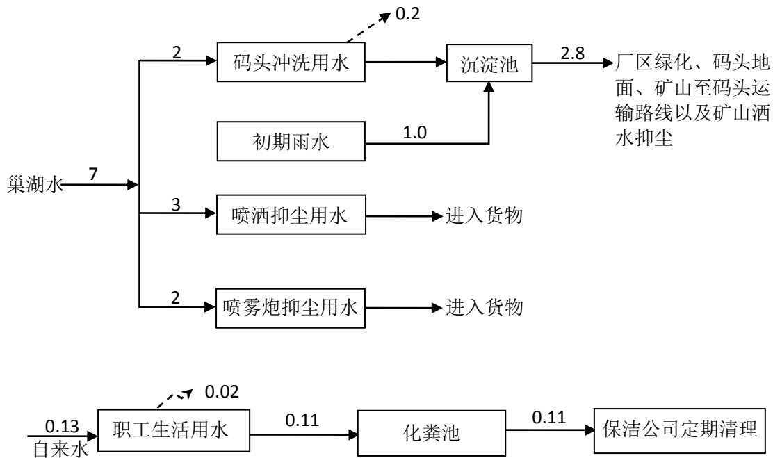
图 3-4 验收期间项目实际水平衡图（单位：m³/d）
